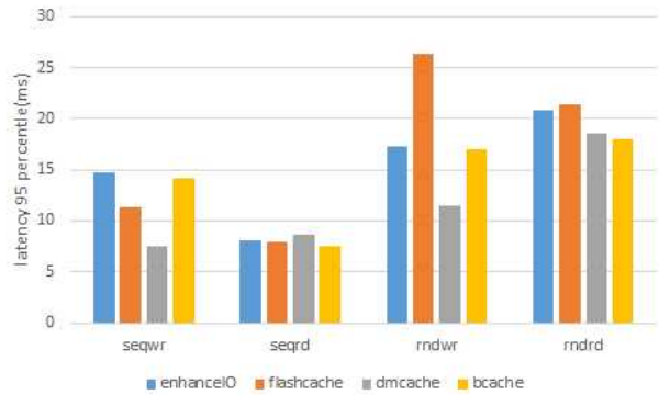
그림 2. 액세스방법에 따른 각 mechanism 지연시간
