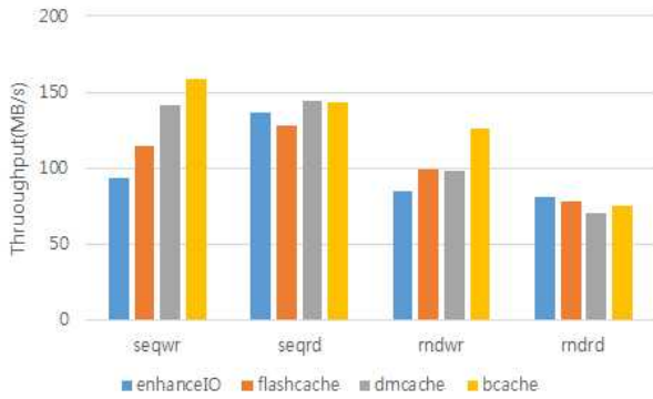
그림 1. 액세스방법에 따른 각 mechanism 처리량(sysbench)
