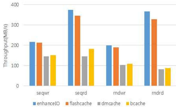
그림 4. 액세스 방법에 따른 각 mechanism 처리량(fio)
